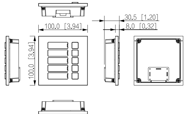
DHI-VTO4103FB-MB5
