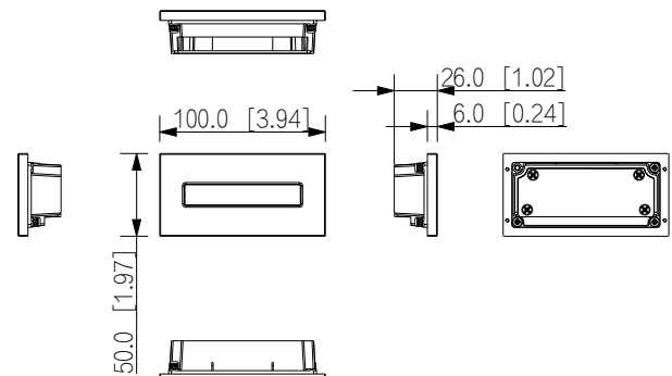
DHI-VTO4103FB-MDB2
