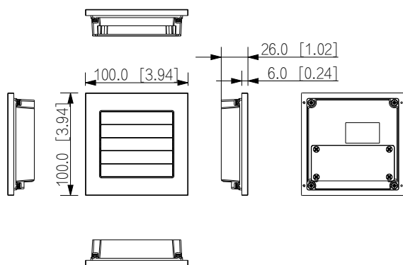
DHI-VTO4103FB-MDB10
