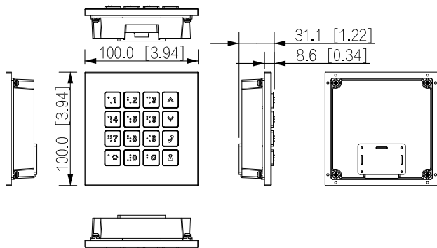
DHI-VTO4202FB-MK
