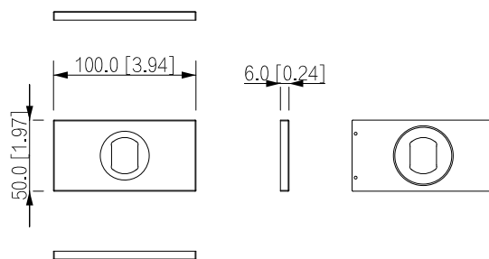
DHI-VTO4202FB-MV
