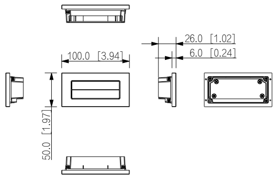
DHI-VTO4202FB-MDB4
