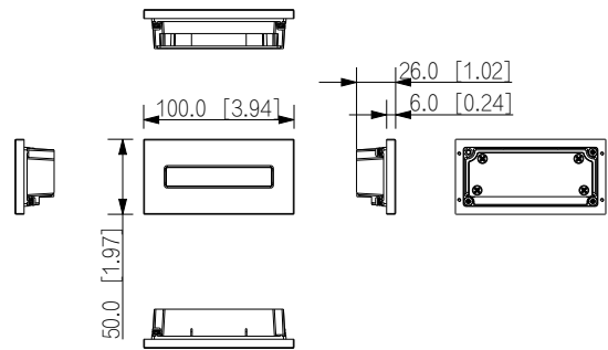
DHI-VTO4202FB-MDB2
