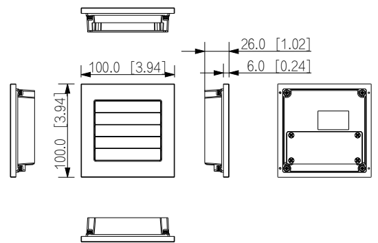
DHI-VTO4202FB-MDB10
