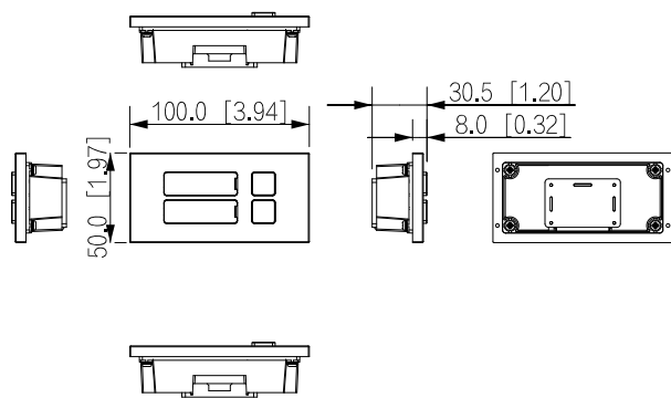
DHI-VTO4202FB-MB2
